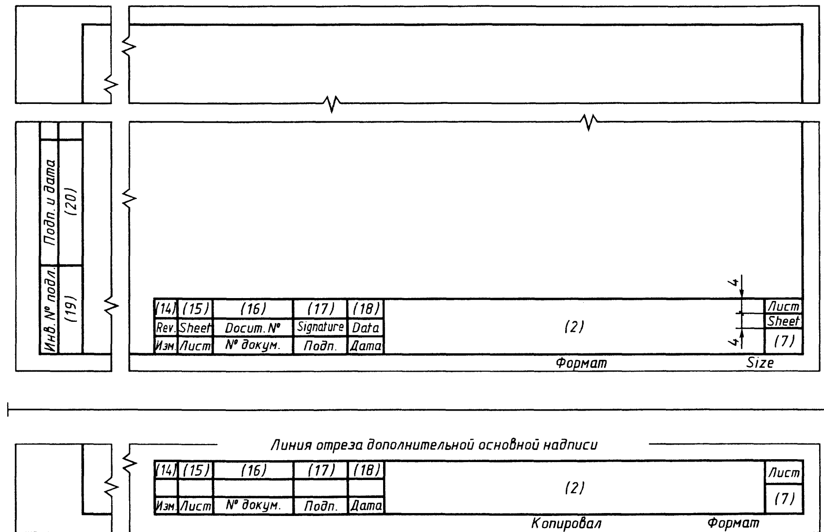
Форма 3 — Основная надпись для текстовых конструкторских документов (последующие листы)
