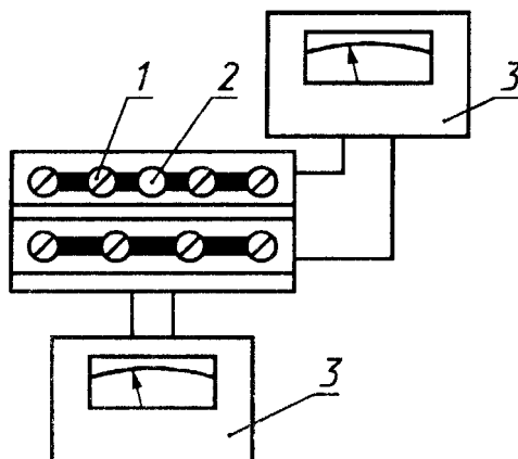
Рисунок 1 — Пример применения клеммы типа КИ-4М Figure 1. An example of using KI-4M type terminals
